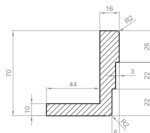
Карниз К2 Р (прямой) Высота карниза 70 мм
