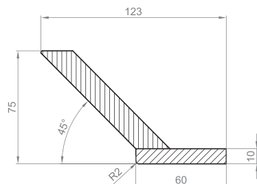
Карниз К0 У (угловой) Угол наклона 45° Высота карниза может изменяться от 30 мм до 150 мм
